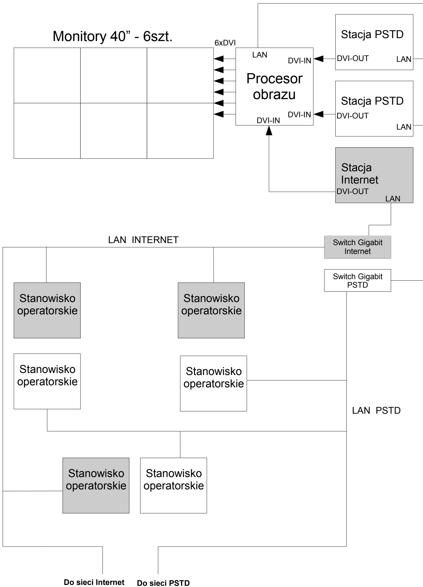
- rys. nr 1: Schemat Blokowy Systemu
