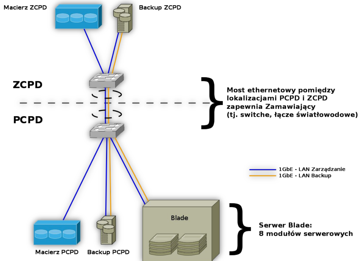
Rys. 3. Schemat wymaganych połączeń Ethernet w ramach SYSTEMU
