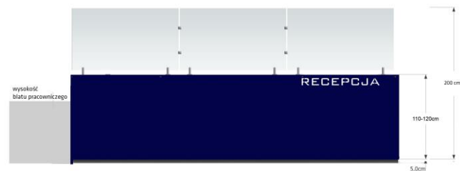
Rys. Widok frontowy (opcja z przeszkleniem)
